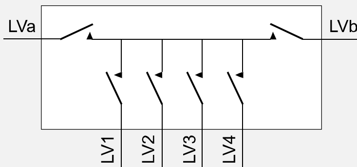
Rysunek 6. Komutator M2770
